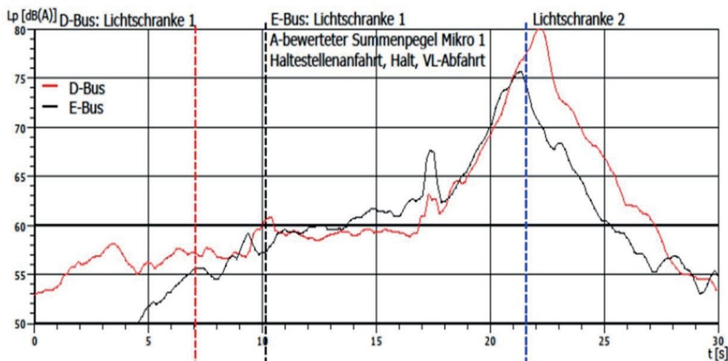
Abbildung 4: Außengeräusch bei Haltestellenanfahrt (A-bewerteter Summenpegel): Vorteile für E-Busse
