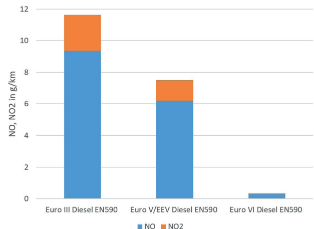
Abbildung 2: Stickoxidemissionen von Solo-Linienbussen unterschiedlicher Grenzwertstufen auf der Landshuter Linie 3
