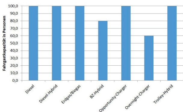
Abbildung 5: Fahrgastkapazität von Solo-Linienbussen nach Antriebssystem
