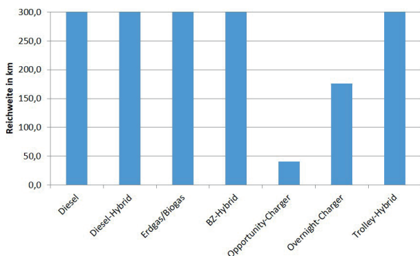
Abbildung 6: Reichweite von Solo-Linienbussen nach Antriebssystem (gefordert: >300 km pro Tag)
